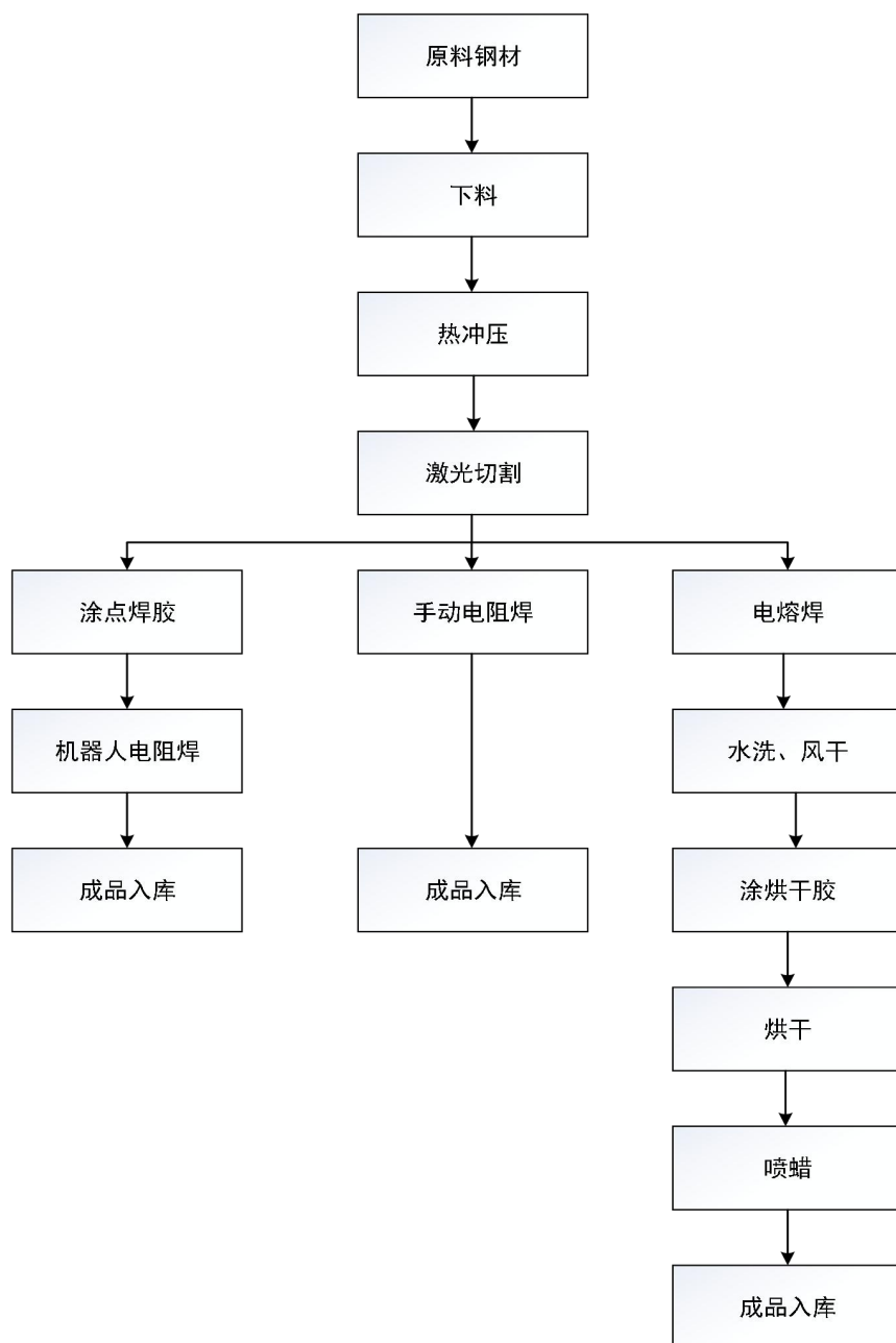
工艺流程图
